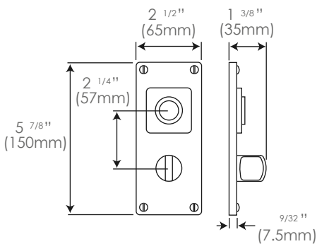
Multipoint Entry FDMP 01 (unsprung)
