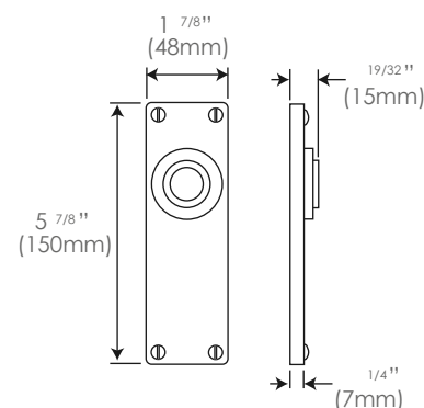
Bathroom FD039 (un-sprung)
