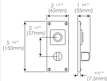
Multipoint Entry FDMP 24 (unsprung)
