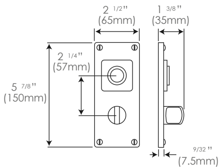
Multipoint Entry FDMP 19 (unsprung)
