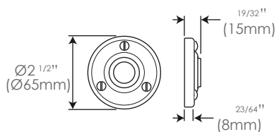
Latch/Passage FD301 (sprung)
