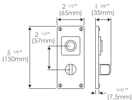
Multipoint Entry FDMP 02 (unsprung)
