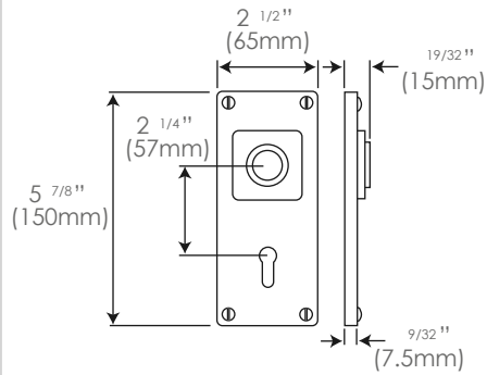
Multipoint Passage FDMP 11 (unsprung)
