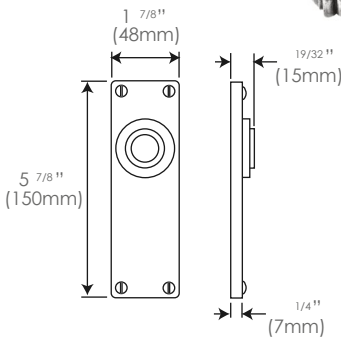
Bathroom FD004 (sprung)
