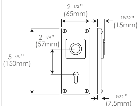
Multipoint Passage FDMP 15 (unsprung)
