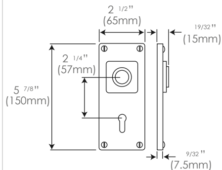
Multipoint Passage FDMP 21 (unsprung)
