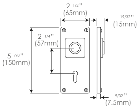
Multipoint Passage FDMP 12 (unsprung)
