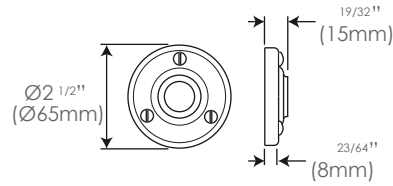
Latch/Passage FD063 (sprung)
