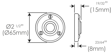
Latch/Passage FD059 (sprung)
