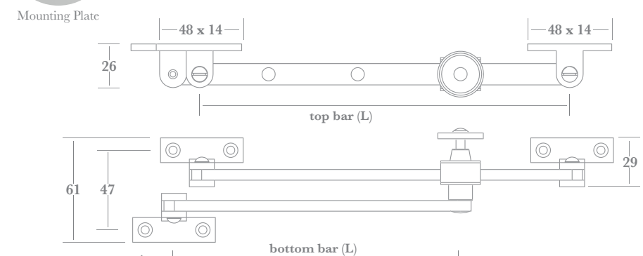
8033 & 8037 INWARD opening windows
