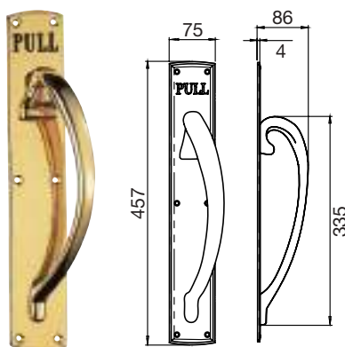
PF104EL Left hand
