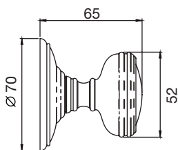
DK34 Porcelain knob face fix Unsprung
