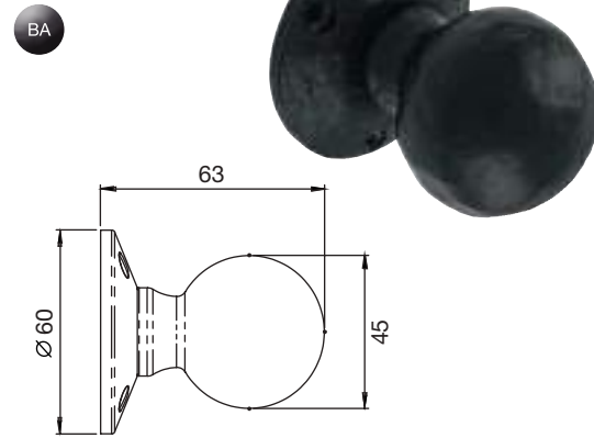
LF5550 Octagonal centre door knob
