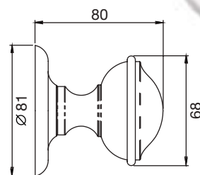
M220 Easy centre door knob
