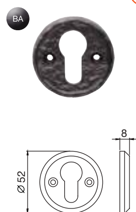
LF5539 Euro escutcheon
