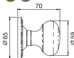
MK001 Oval mortice knob Unsprung
