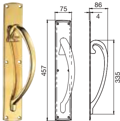
PF101L Left hand
