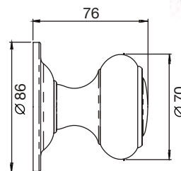
M60 Round centre door knob
