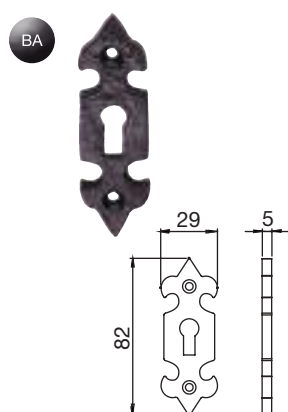
LF5532 Lock Fleur de Lys escutcheon
