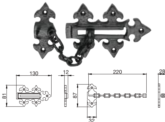
LF5536 Door chain
