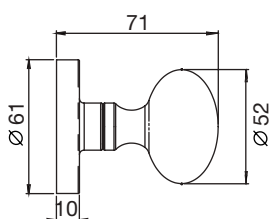
M35US Mushroom mortice knob Unsprung
