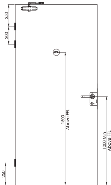
FDPC3 & FDPR3 Lever Lock
